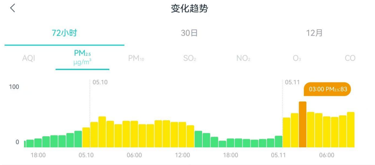
图 3 5 月 10 日—11 日 PM 2.5 浓度变化趋势
