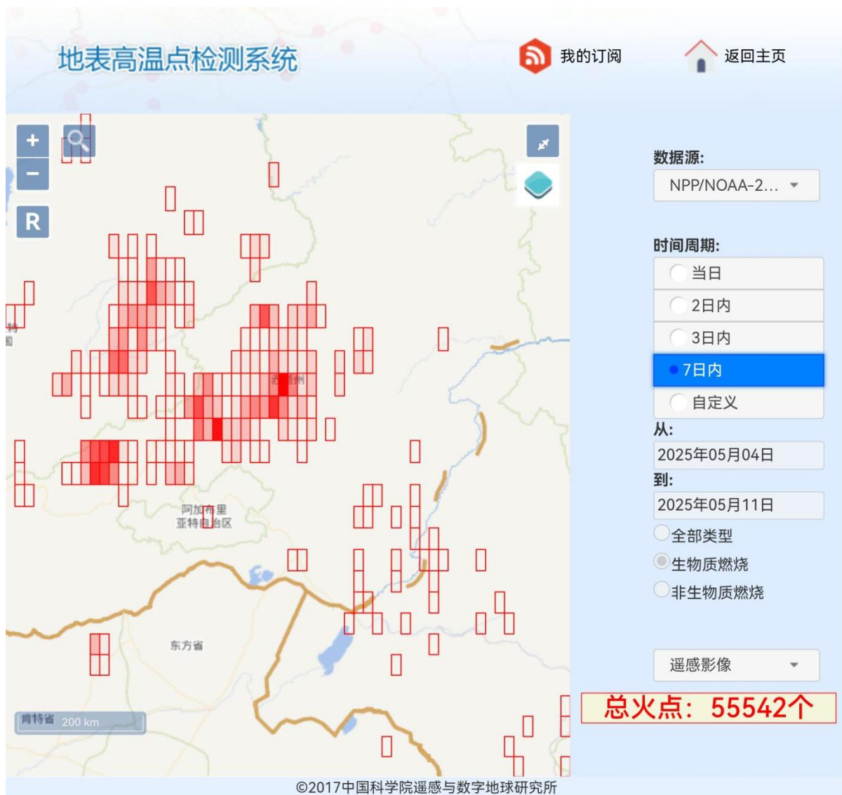
图1 近七日内卫星遥感火点监测影像图
