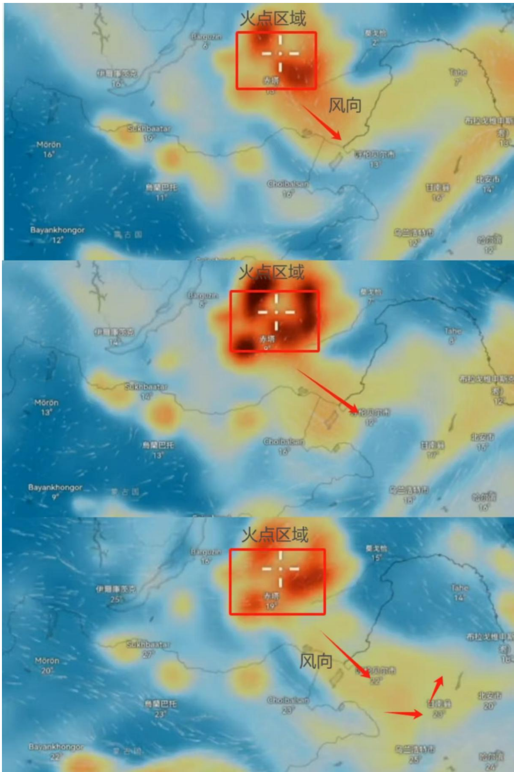
图 2 5 月 10 日—12 日烟尘传输过程影像图
